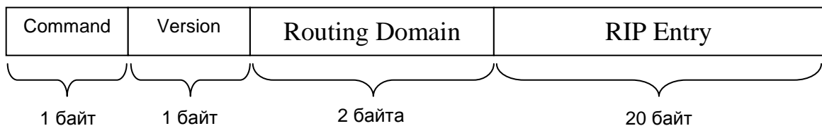
Рис. 3.20. Формат RIP-пакета
