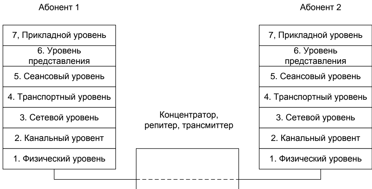
Рис.1.10. Функции концентраторов, репитеров в модели ВОС
