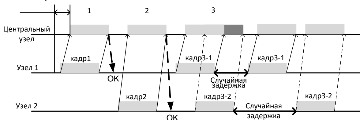
Рис. 2.3. Передача кадров по алгоритму ALOHA
