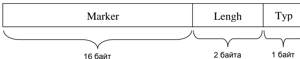
Рис. 3.32. Формат заголовка BGP-сообщения
