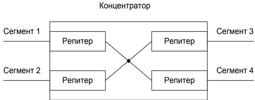
Рис.1.9. Структура концентратора
