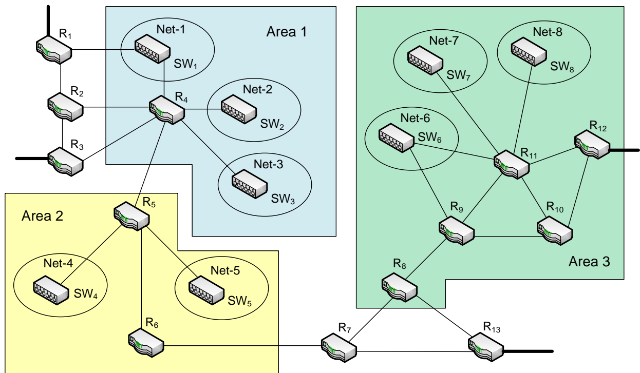
Рис. 3.24. Выделенные зоны при использовании OSPF
