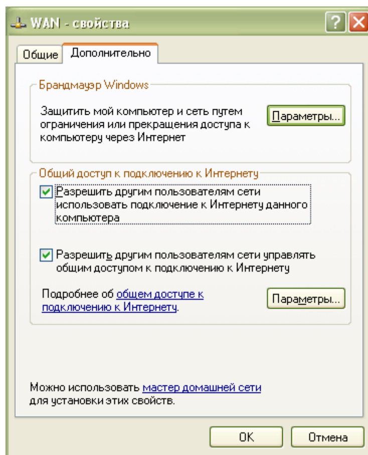
Рис. 3.39. Включение NAT в ОС Windows
