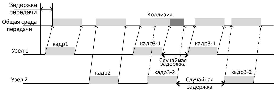
Рис. 2.4. Передача кадров по методу доступа CSMA/CD
