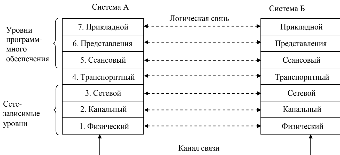
Рис. 1.7. Структура эталонной модели ВОС
