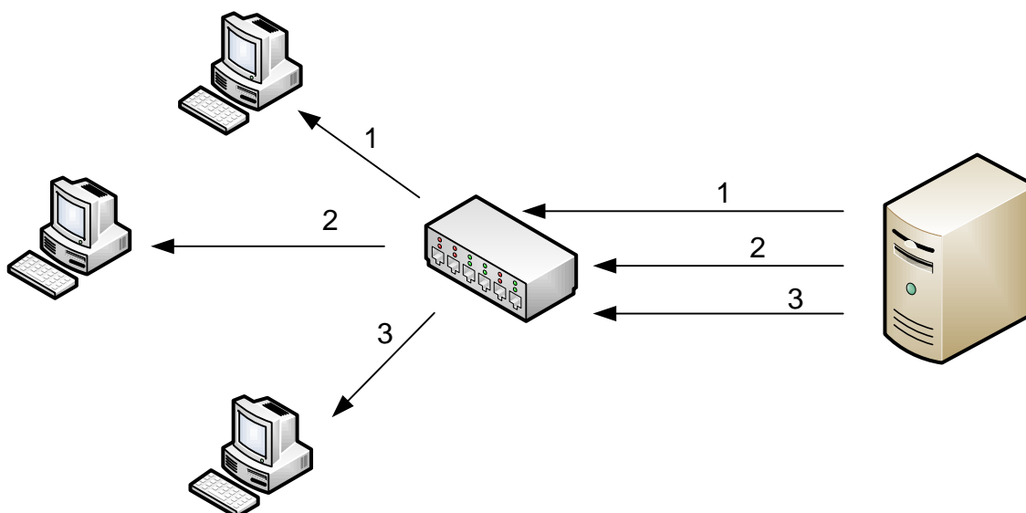
Рис. 3.33. Принцип организации unicast-вещания сервера с тремя клиентами
