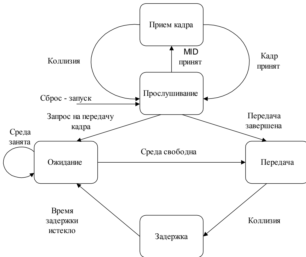
Рис. 2.5. Алгоритм CSMA/CD
